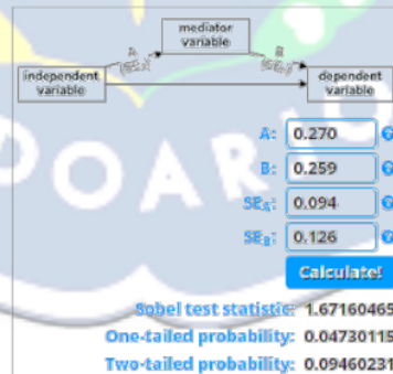
Gambar 3.1 Uji Sobel X1
