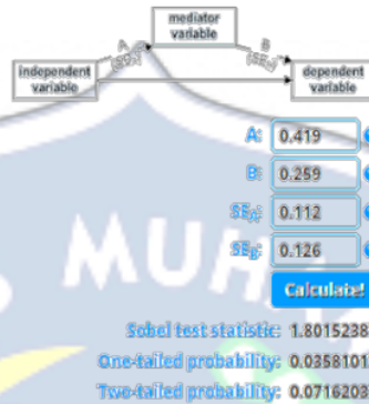
Gambar 3.2 Uji Sobel X2
