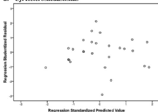
Gambar 3. Uji Heterokedastisitas
