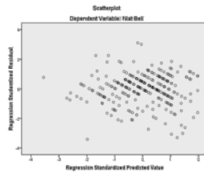
Gambar 3.1 Hasil Pengujian Heteroskedastisitas
