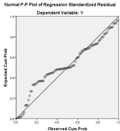
Gambar 3.1 Hasil Uji Normalitas
