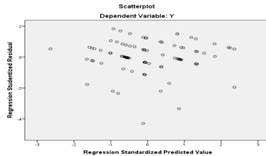
Gambar 3.2 Hasil uji Heterokedastisitas
